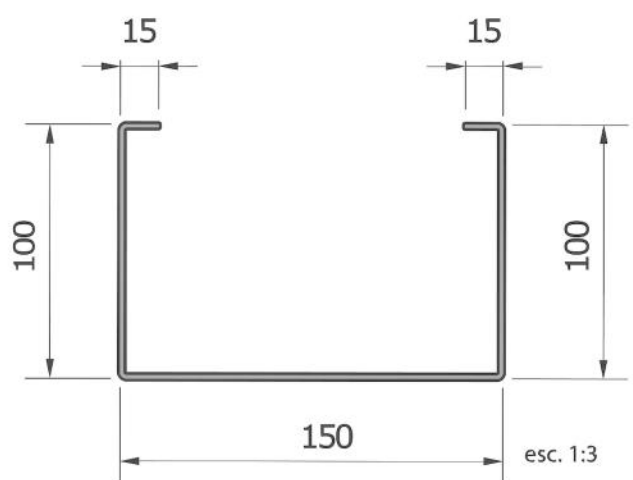
T128 - Viga de cima sem batente
