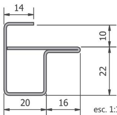
T35 - Perfil F amassado
