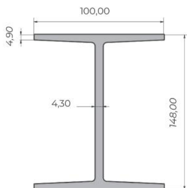
Viga W cód. 2507
