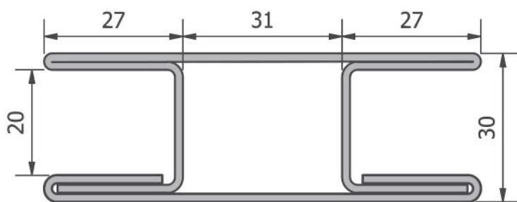
T27 - Perfil H móvel
