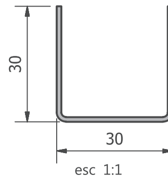
T80 - Perfil U serralheiro
