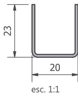
T81 - Perfil U serralheiro
