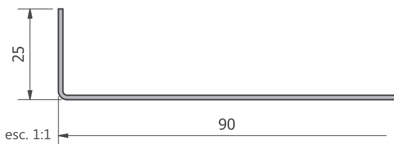
T22 - Perfil L
