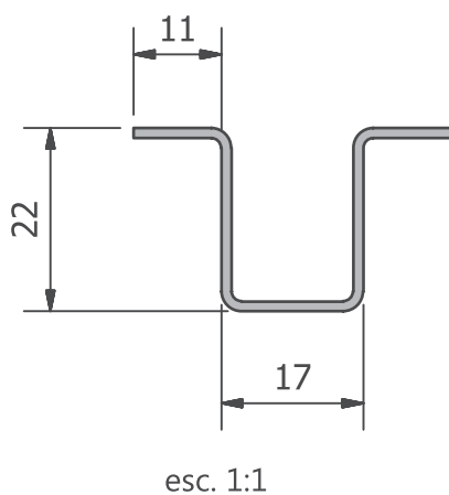
T26 - Trilho inferior
