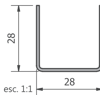
T7 - Perfil U
